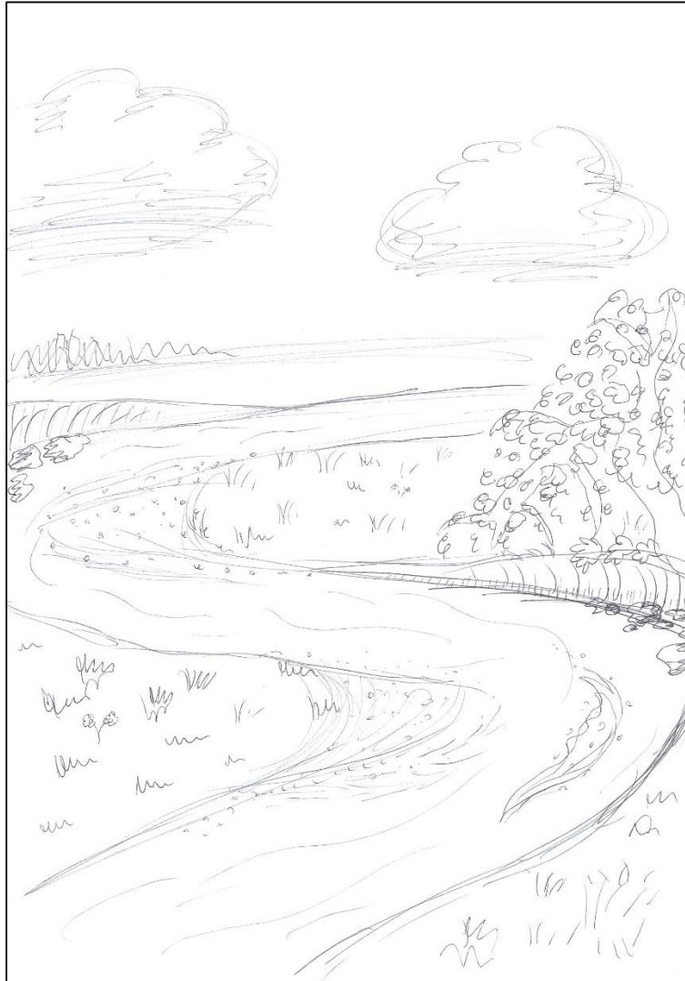
Rzeka meandrująca
