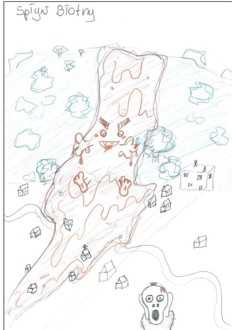
Spływ błotny
