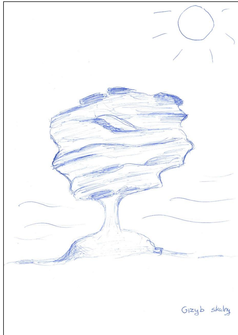
Grzyb skalny
