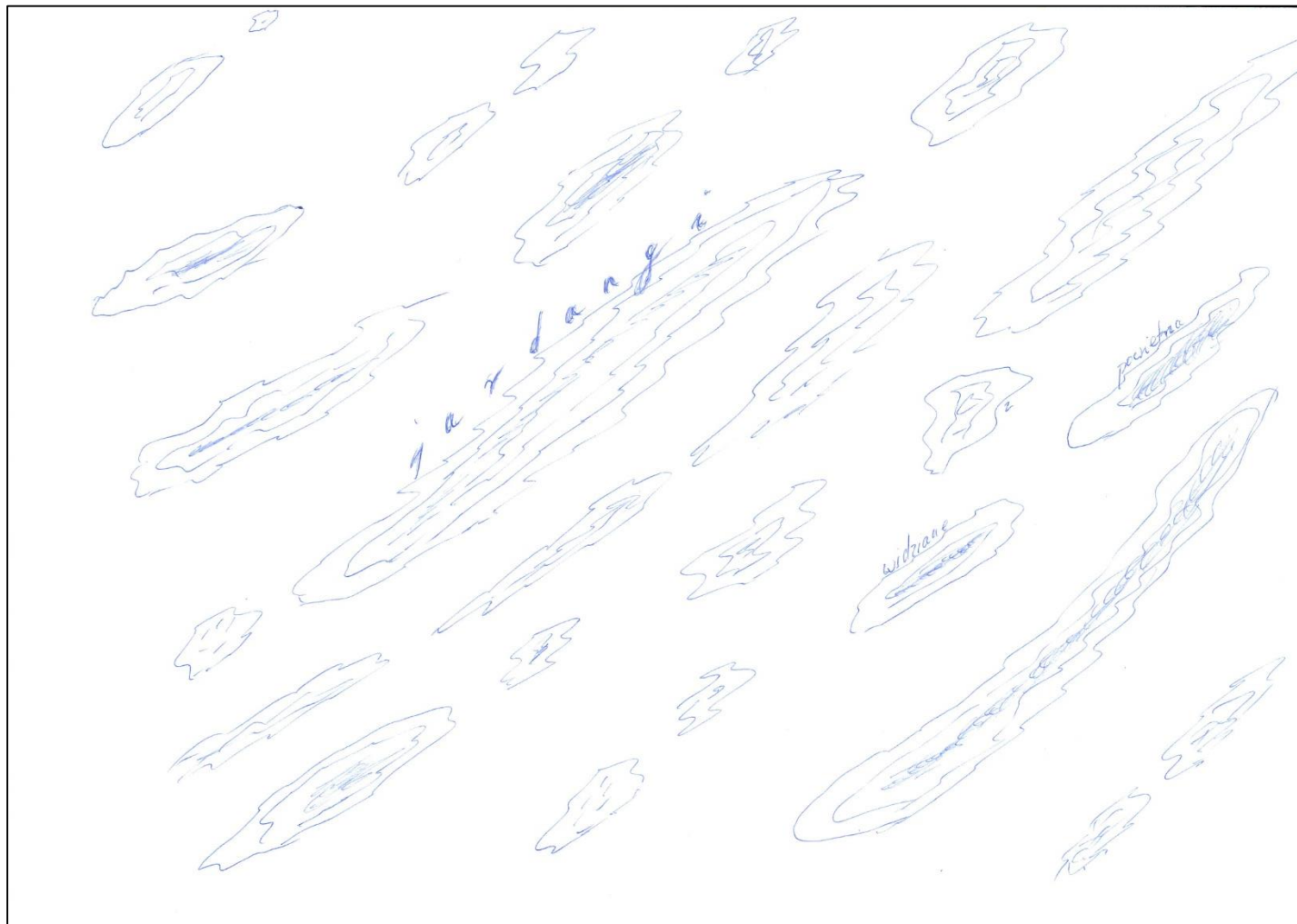
Jardangi
