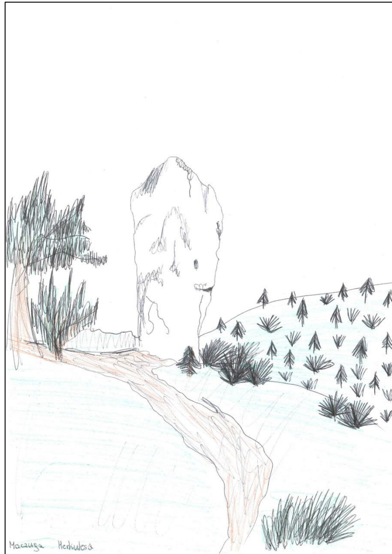
Ostaniec
