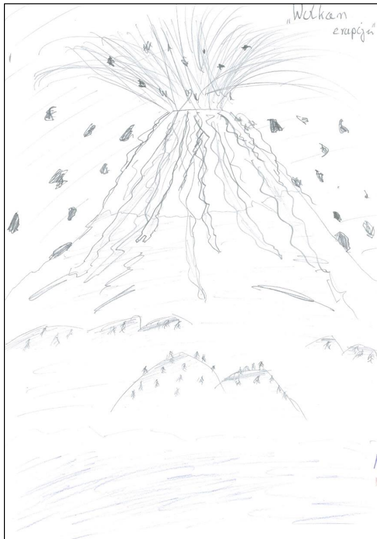
Wulkan
